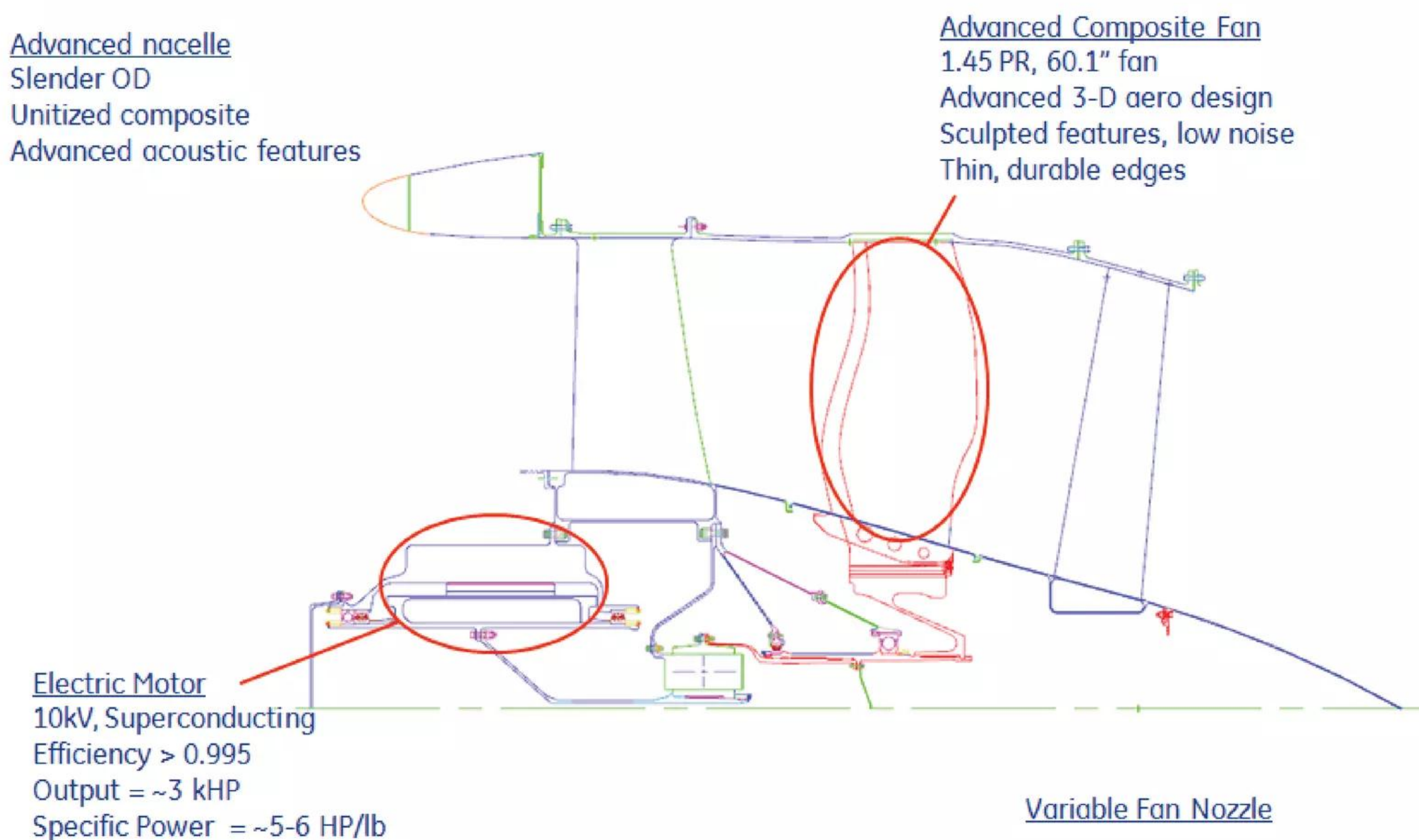
Figure 5 - LNG+2045GT+SOFC+DF+BLI (Fuselage Fan)
